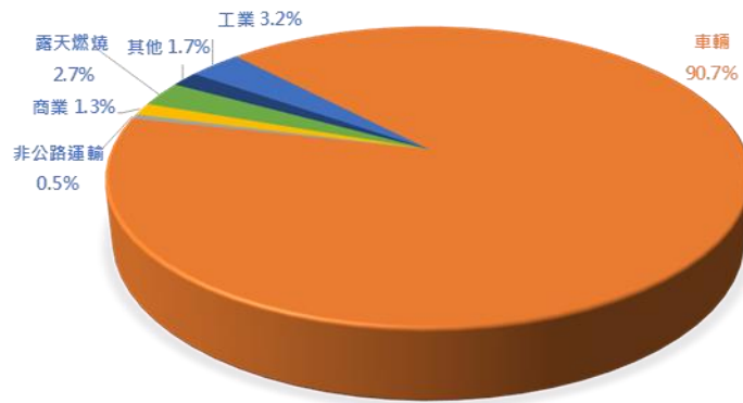
圖 3.2-4 NO x (氮氧化物)排放比例
