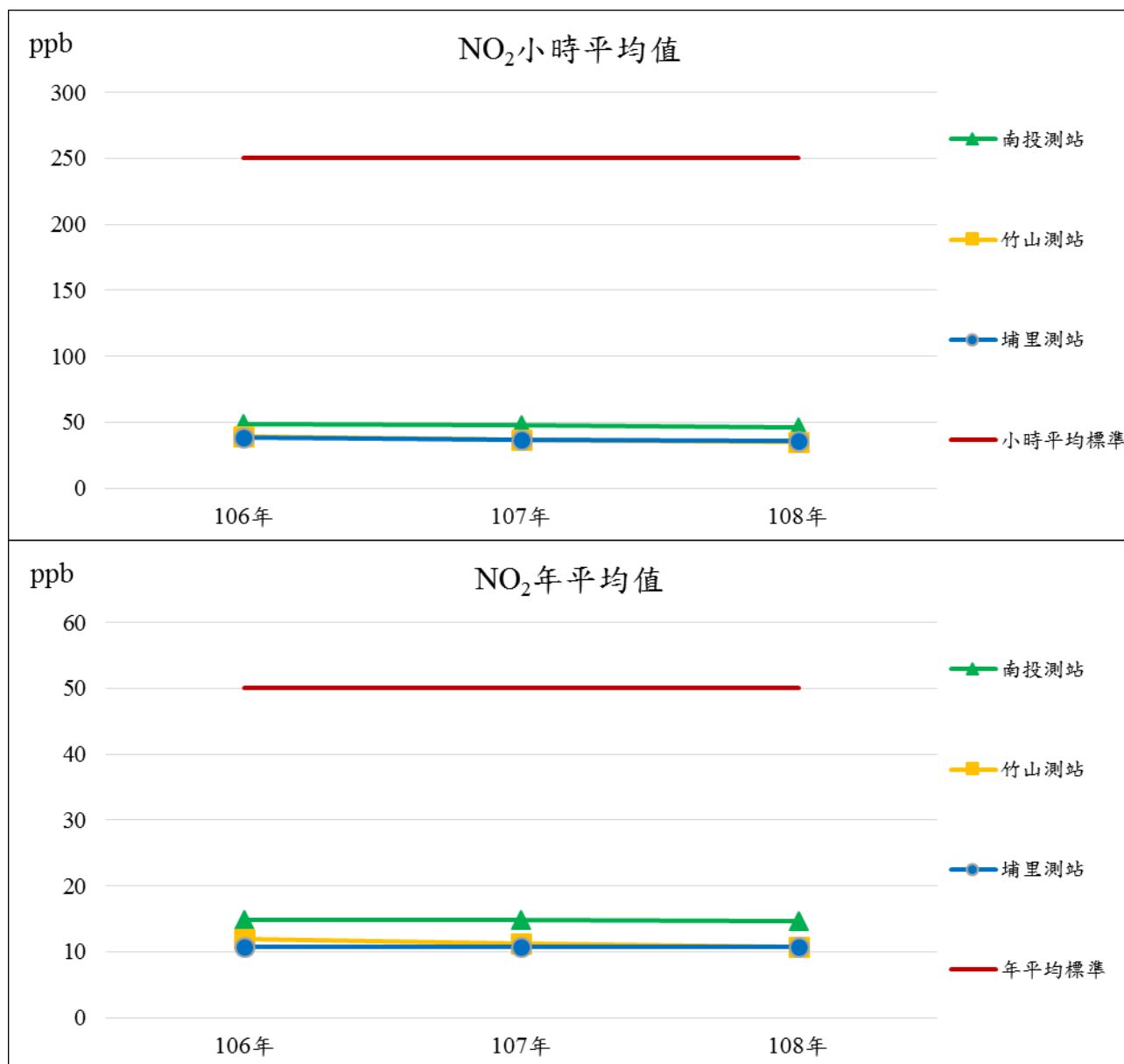
圖 3.1-5 南投縣 106 - 108 年年二氧化氮(NO 2 )濃度趨勢圖
