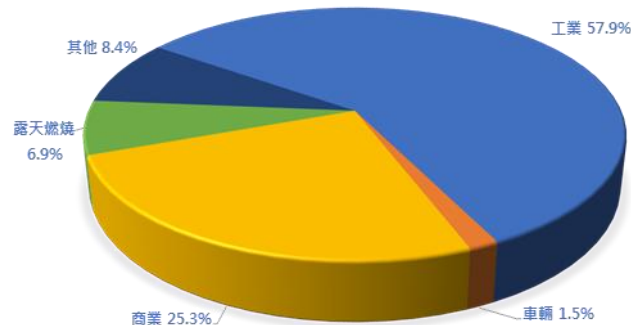
圖 3.2-3 SO x (硫氧化物)排放比例
