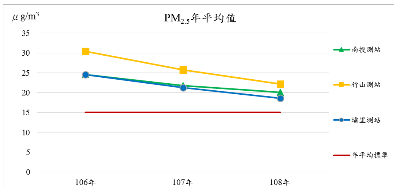
圖 3.1-3 南投縣 106 - 108 年年細懸浮微粒(PM 2.5 )濃度趨勢圖
