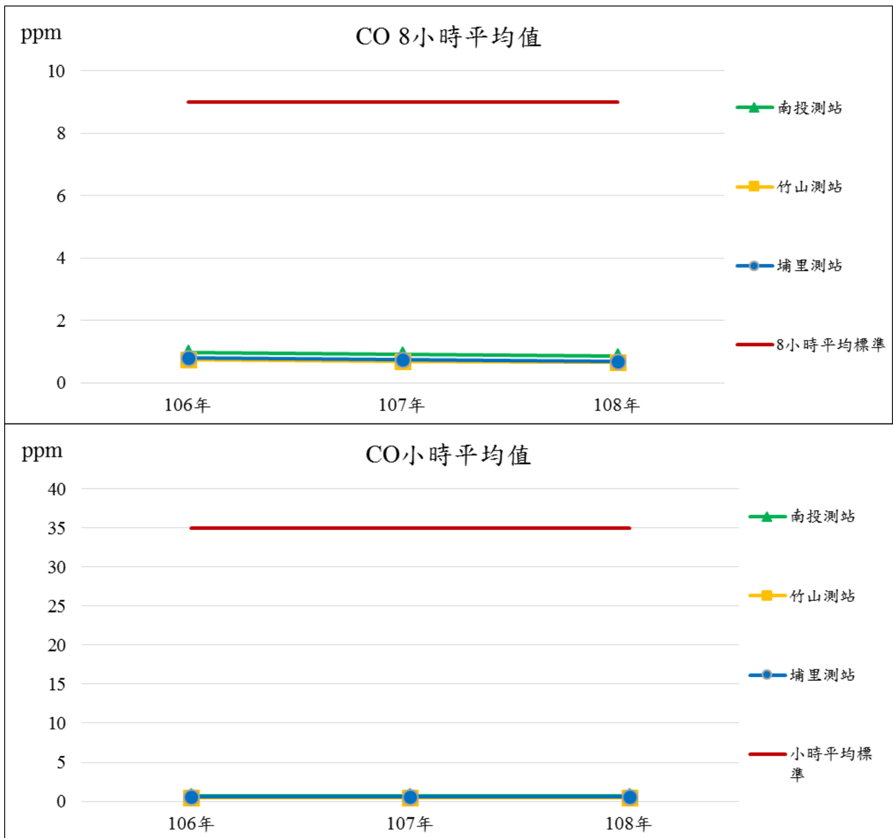
圖 3.1-6 南投縣 106 - 108 年年一氧化碳(CO)濃度趨勢圖
