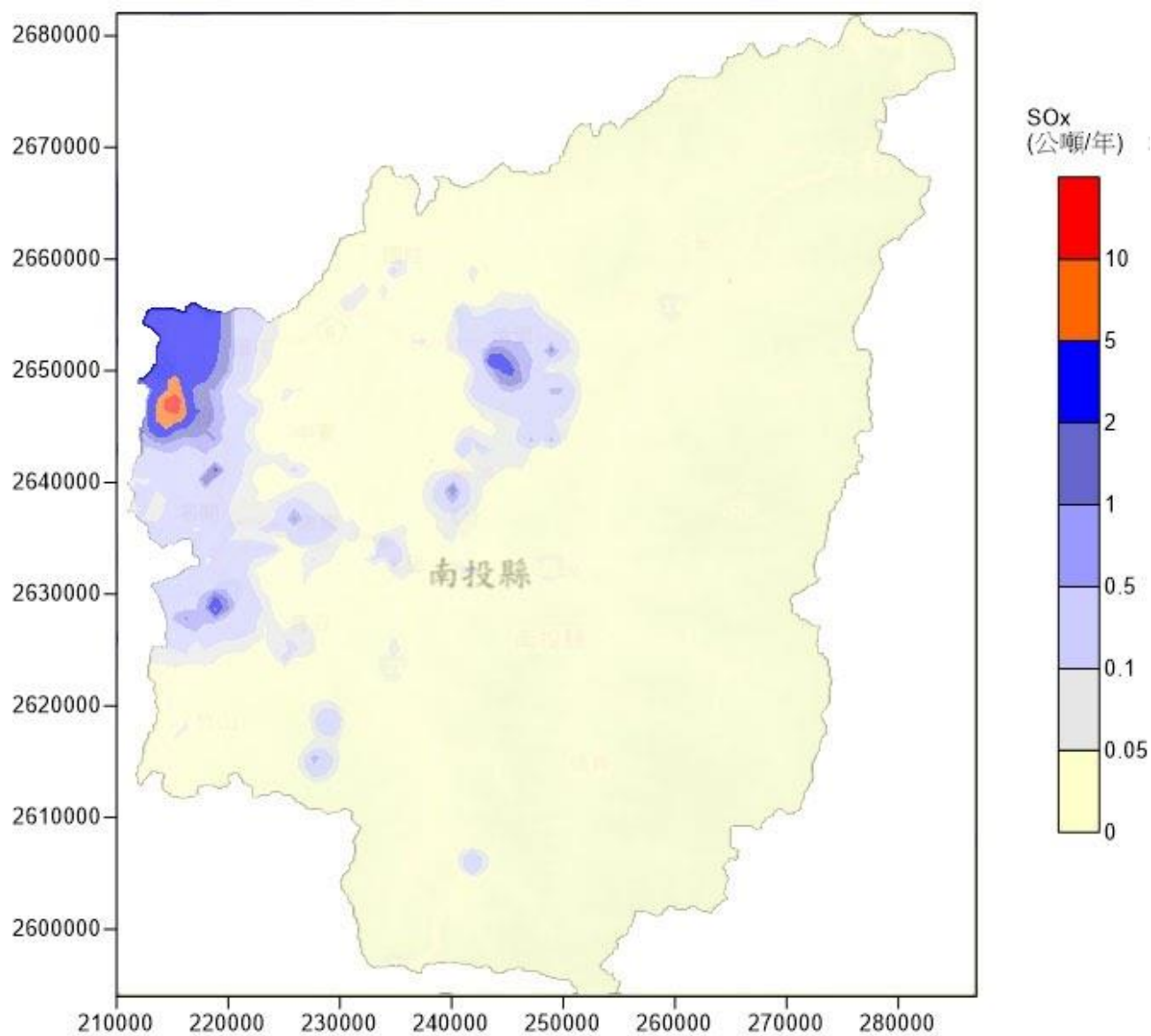
圖 3.2-7 南投縣硫氧化物（SO x ）排放地圖
