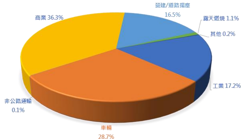
圖 3.2-5 NMHC(非甲烷碳氫化合物)排放比例
