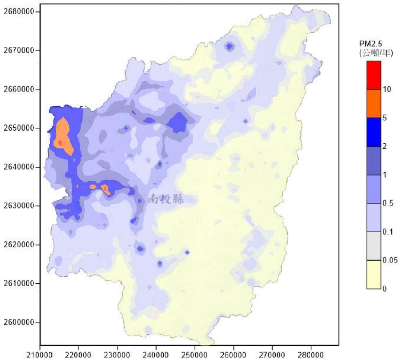
圖 3.2-6 南投縣細懸浮微粒 ( PM_{2.5} ) 排放地圖
