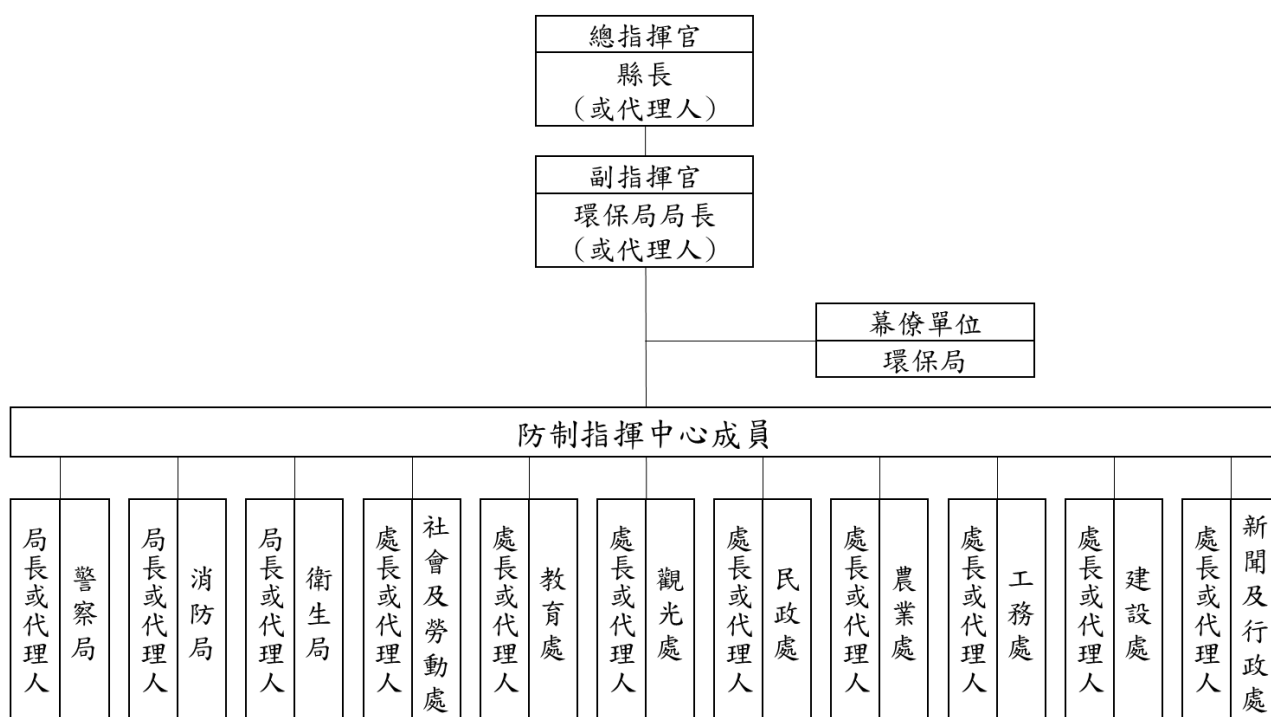
圖 8.1-1 南投縣空氣污染防制計畫分工組織架構圖
