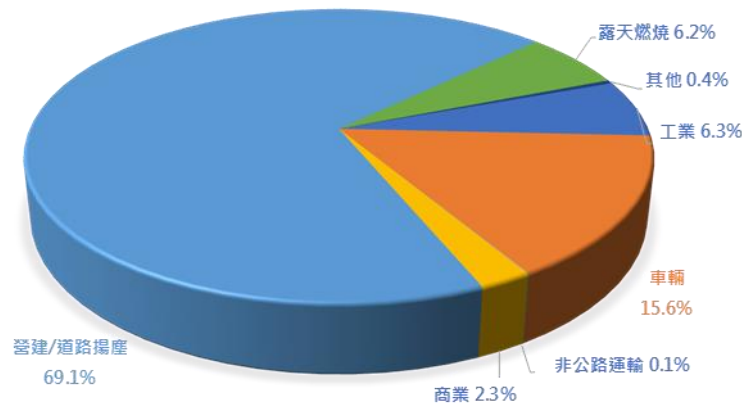
圖 3.2-1 PM 10 (懸浮微粒)排放比例
