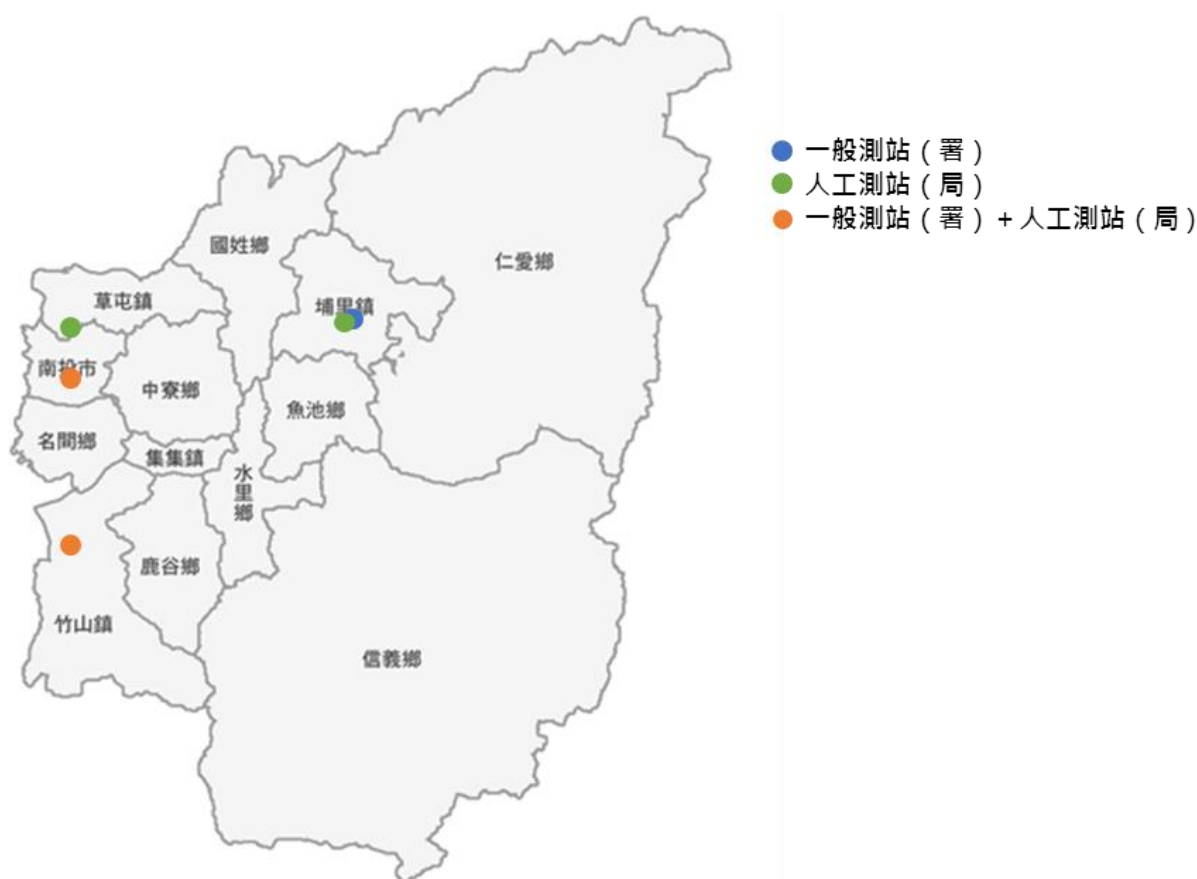
圖 3.1-1 南投縣空氣品質監測站位置圖
