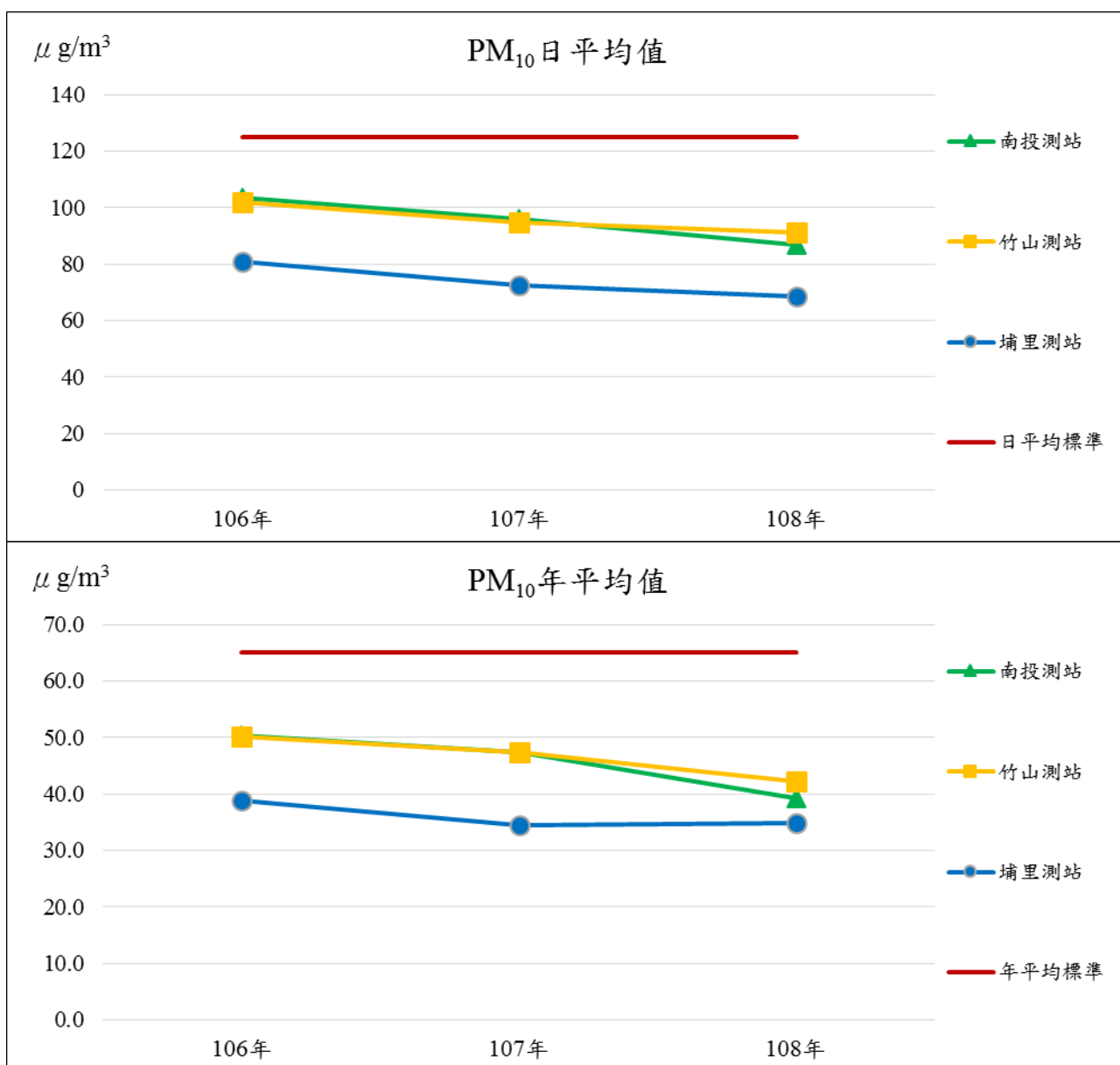
圖 3.1-2 南投縣 106 - 108 年年懸浮微粒(PM 10 )濃度趨勢圖
