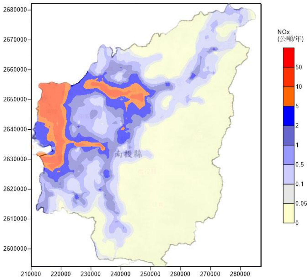
圖 3.2-8 南投縣氮氧化物 (NO x ) 排放地圖
