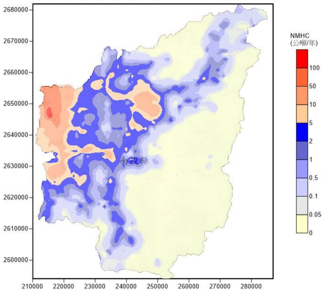
圖 3.2-9 南投縣揮發性有機物（VOCs）排放地圖
