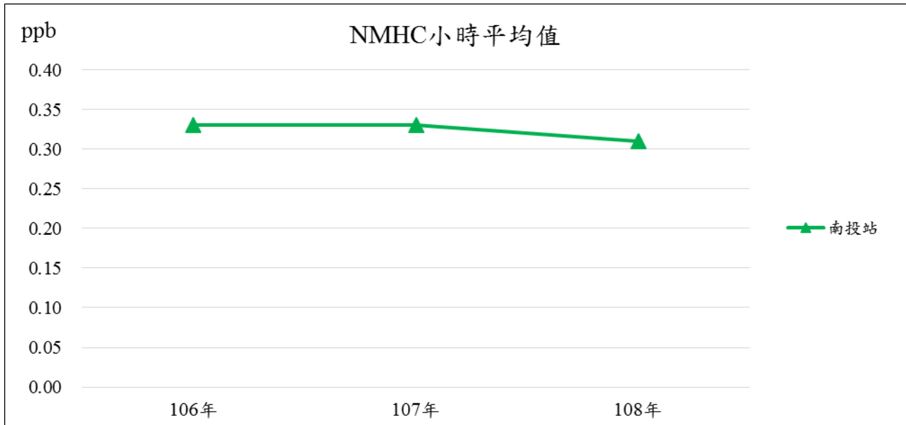
圖 3.1-8 南投縣 106 - 108 年非甲烷碳氫化合物(NMHC)濃度趨勢圖
