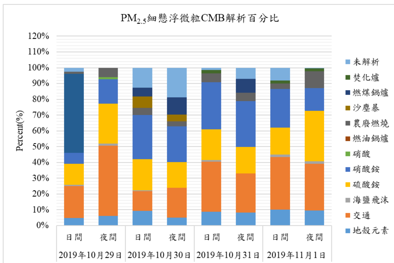
圖 3.3-3 CMB 模式解析南投縣竹山鎮 PM 2.5 的污染源貢獻量分佈圖
