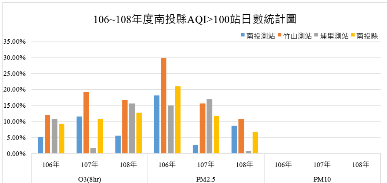
圖 3.1-10 106 – 108 年度南投縣 AQI>100 站日數統計圖
