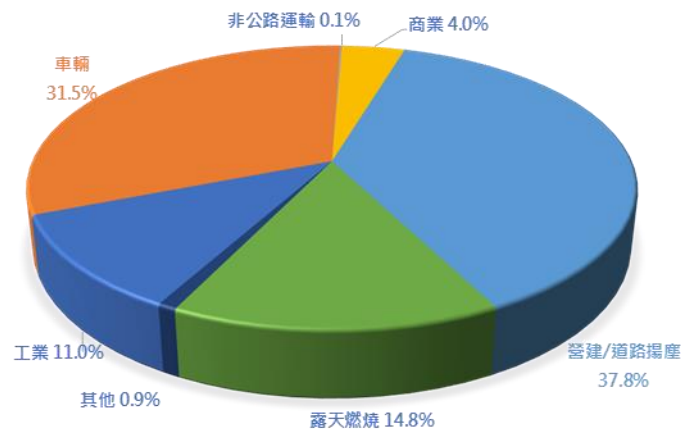
圖 3.2-2 PM 2.5 (細懸浮微粒)排放比例
