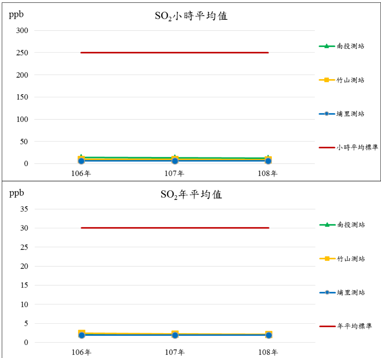
圖 3.1-4 南投縣 106 - 108 年年二氧化硫(SO 2 )濃度趨勢圖
