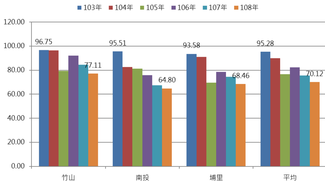
圖 3.3-1 南投縣 103 年~108 年 AQI 年平均值
