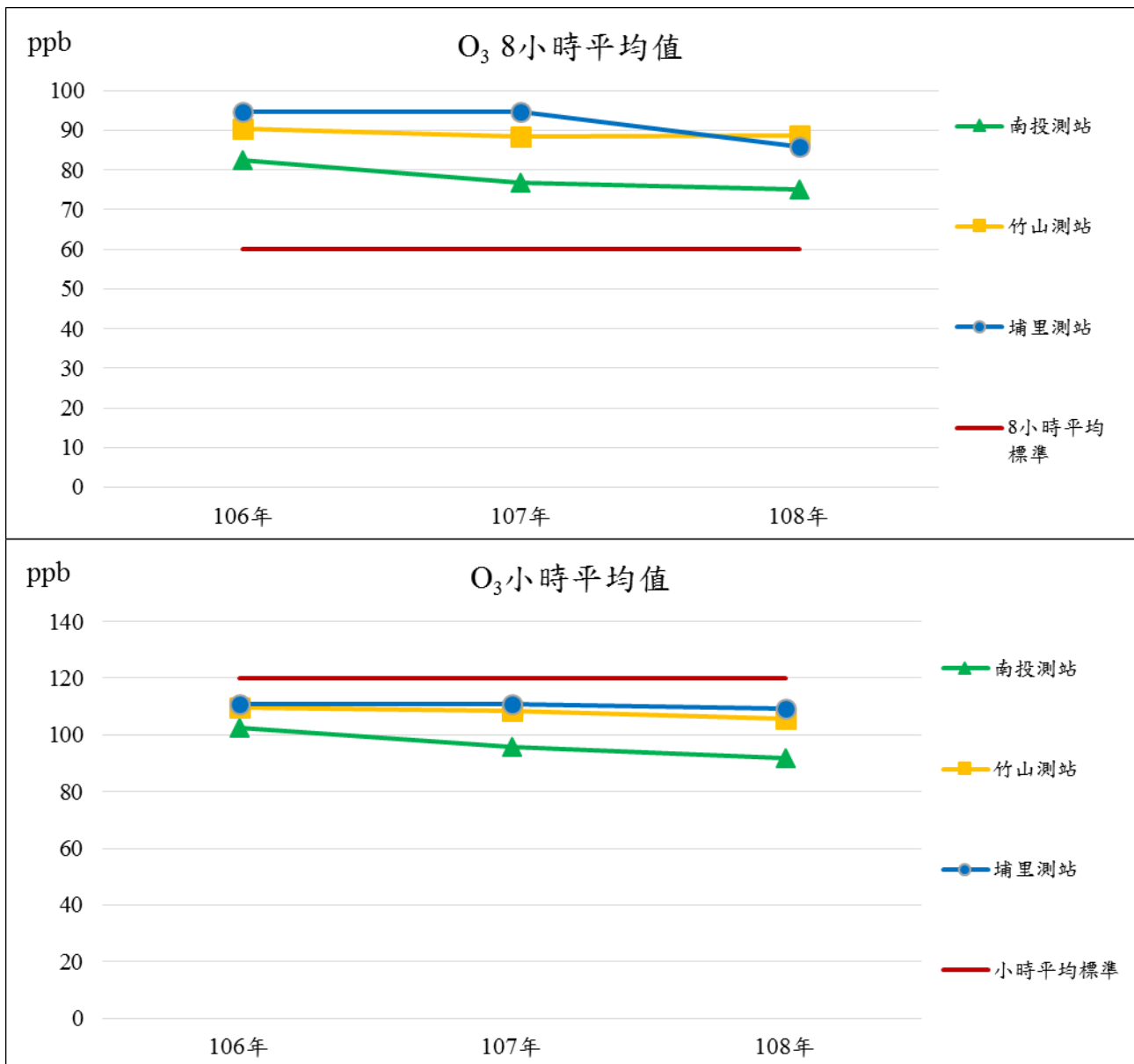
圖 3.1-7 南投縣 106 - 108 年臭氧(O 3 )濃度趨勢圖
