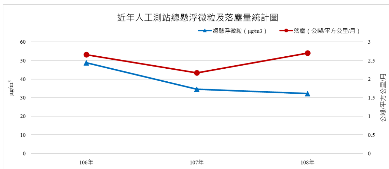
圖 3.1-9 南投縣近年人工測站總懸浮微粒及落塵統計分析圖
